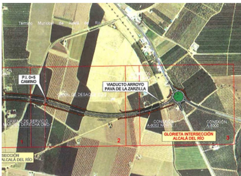
Nueva construcción del ramal que conectará Alcalá del Río con Sevilla
